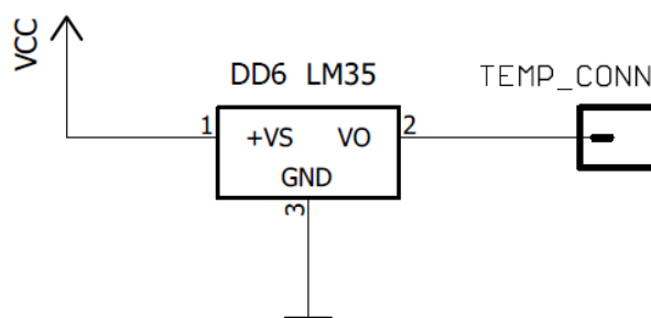
Рис.3.13. Схема підключення датчика LM35
